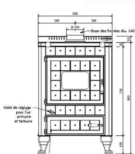
Volet de réglage pour l'air primaire et tertiaire Vanne supplémentaire pour l'air primaire dans la porte du cendrier VUE AVANT H 900 mm
