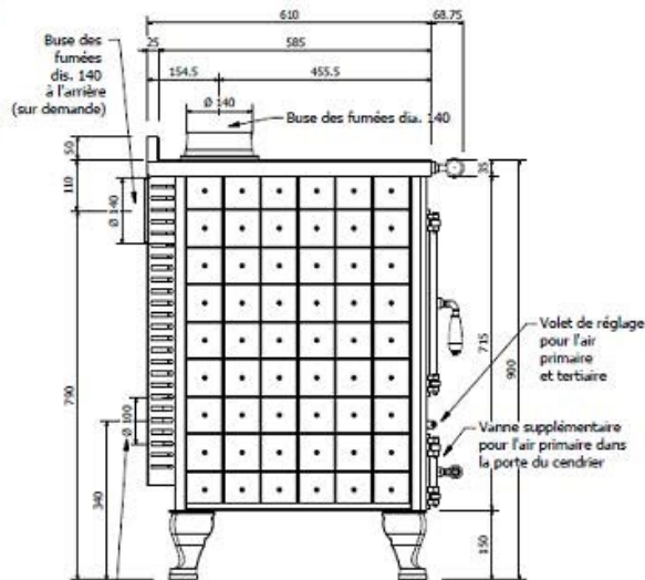
Buse des fumées dia. 140 à l'arrière (sur demande) Buse des fumées dia. 140 Volet de réglage pour l'air primaire et tertiaire Vanne supplémentaire pour l'air primaire dans la porte du cendrier Buse entrée de l'air primaire et tertiaire VUE LATÉRALE H 900 mm
